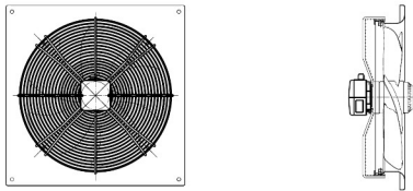
Rys. 1. Montaż wentylatora WAX.
